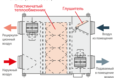
Схема (SAF1000E6)
