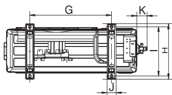
Наружный блок
